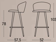
TABURETE ALTO SEDA 7532 ASIENTO Y RESPALDO TAPIZADO PATA REDONDA MADERA CÓNICA
