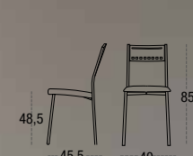
SILLA ALOHA 45 ASIENTO TAPIZADO TUBO CUADRADO METÁLICO DE 20
