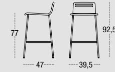
TABURETE ALTO DURERO 7551 CARCASA MADERA PATA CUADRADA METÁLICA DE 18
