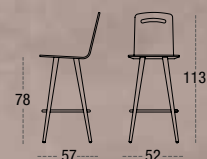
TABURETE ALTO DURBAN 7511 CARCASA MADERA PATA CUADRADA MADERA DESPUNTADA
