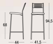
TABURETE MEDIO FORMENTERA 65 ASIENTO TAPIZADO TUBO CUADRADO METÁLICO DE 20
