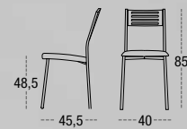
SILLA FORMENTERA 45 ASIENTO TAPIZADO TUBO CUADRADO METÁLICO DE 20
