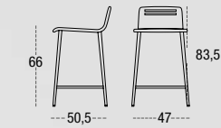
TABURETE MEDIO DURERO 6552 CARCASA MADERA PATA CUADRADA MADERA DESPUNTADA
