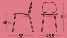
SILLA NIZA ASIENTO Y RESPALDO MADERA FRESNO CHASIS REDONDO METÁLICO Ø 22
