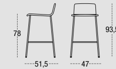
TABURETE ALTO DURERO 7552 CARCASA TAPIZADA PATA CUADRADA MADERA DESPUNTADA
