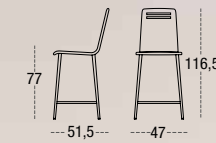
TABURETE ALTO BELICE 7542 CARCASA MADERA PATA CUADRADA MADERA DESPUNTADA
