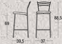
TABURETE MEDIO MARTA 65 ASIENTO TAPIZADO TUBO REDONDO METÁLICO Ø 25
