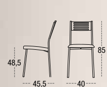
SILLA FORMENTERA 45 ASIENTO TAPIZADO TUBO CUADRADO METÁLICO DE 20
