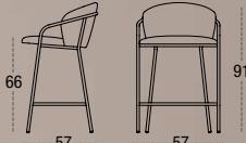
TABURETE MEDIO SEDA 6530 ASIENTO Y RESPALDO TAPIZADO TUBO REDONDO METALICO Ø18
