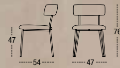
SILLA LOLA ASIENTO Y RESPALDO TAPIZADO TUBO REDONDO METÁLICO Ø18
