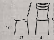
SILLA MARTA 45 ASIENTO TAPIZADO TUBO REDONDO METÁLICO Ø 25
