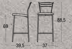
TABURETE MEDIO MARTA 65 ASIENTO TAPIZADO TUBO REDONDO METÁLICO Ø 25
