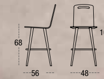
TABURETE MEDIO DURBAN 6511 CARCASA MADERA PATA CUADRADA MADERA DESPUNTADA
