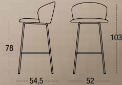
TABURETE ALTO SEDA 7533 ASIENTO Y RESPALDO TAPIZADO PATA REDONDA METÁLICA Ø18
