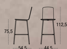
TABURETE ALTO DURBAN 7513 CARCASA TAPIZADA PATA REDONDA METÁLICA Ø 18
