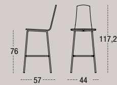
TABURETE ALTO BONN 7503 CARCASA TAPIZADA PATA REDONDA METÁLICA Ø18
