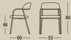
SILLÓN SUPRA ASIENTO Y RESPALDO TAPIZADO TUBO REDONDO METÁLICO Ø20
