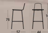
TABURETE ALTO NEUSS 7523 CARCASA TAPIZADA PATA REDONDA METÁLICA Ø 18
