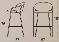
TABURETE ALTO SEDA 7530 ASIENTO Y RESPALDO TAPIZADO TUBO REDONDO METÁLICO Ø18
