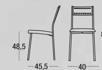
SILLA ALOHA 45 ASIENTO TAPIZADO TUBO CUADRADO METÁLICO DE 20
