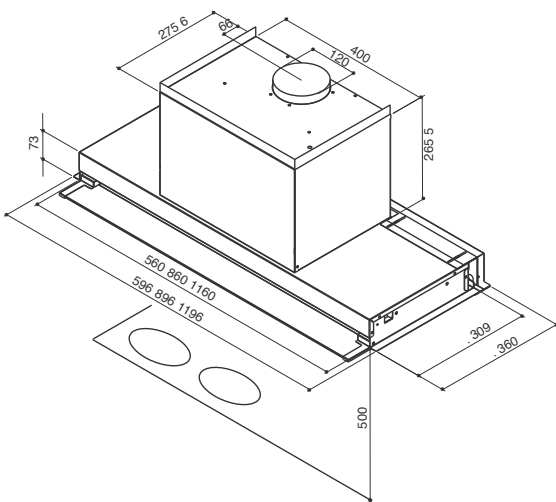
Distancia aconsejada desde la zona de cocción 50 cm.
