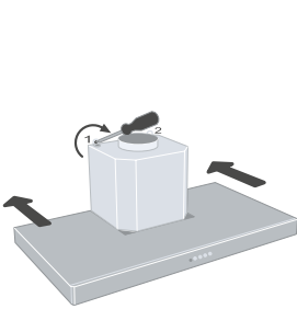
Cuelgue la campana
