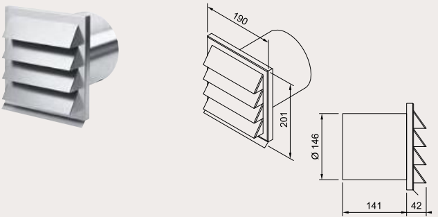
Salida de humos exterior con rejilla
