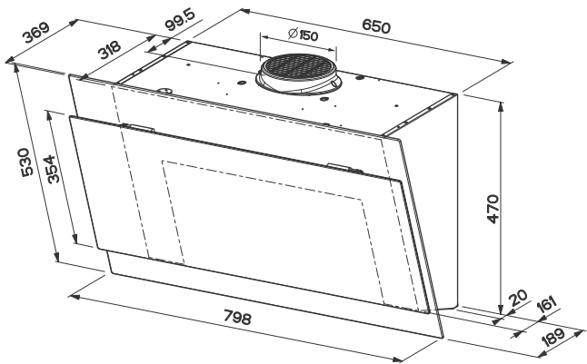
Distancia aconsejada desde la zona de cocción 45 cm.
