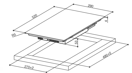
INSTALACIÓN SOBRE ENCIMERA
