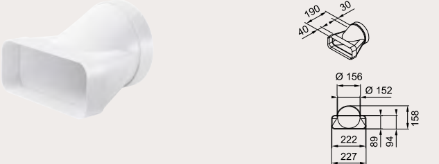
Extremo de tubo
