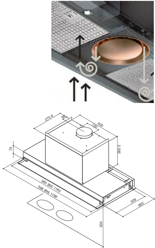
Distancia aconsejada desde la zona de cocción 50 cm.
