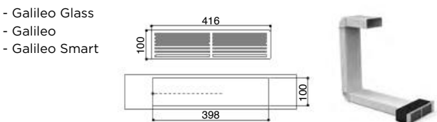
Filtro cerámico incluido en el kit
