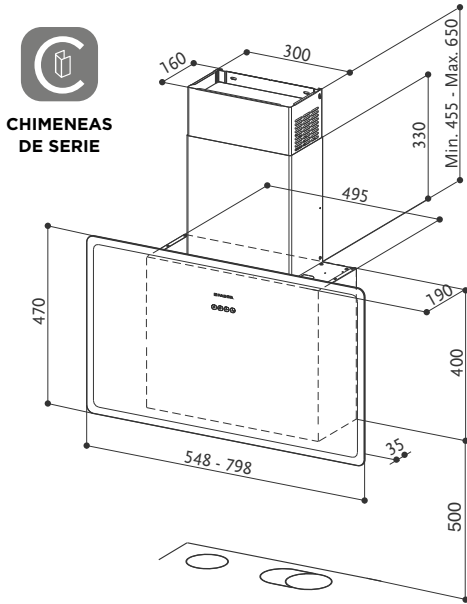
Distancia aconsejada desde la zona de cocción 50 cm.
