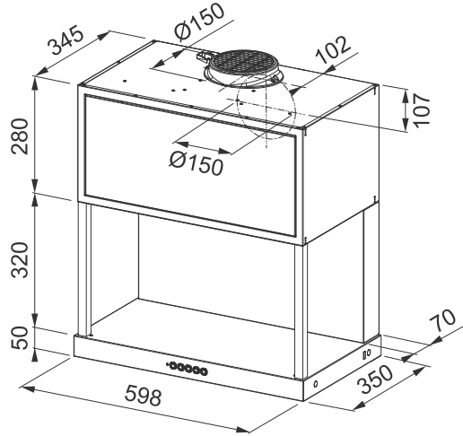
MÓDULO DE CAMPANA
