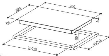
INSTALACIÓN SOBRE ENCIMERA
