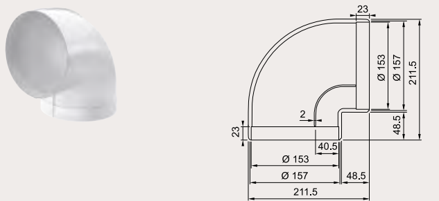
Codo de 90° para tubo redondo 150
