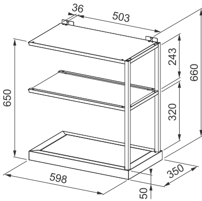
MODULO DE ESTANTERÍA
