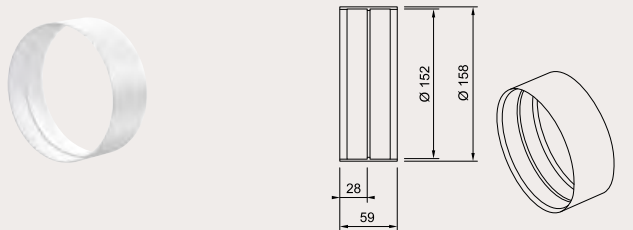
Conector para tubo redondo
