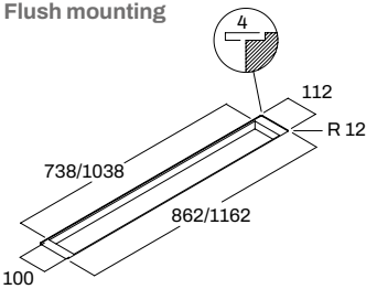
Montaje enrasado Flush mounting
