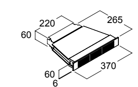
Kit rejilla de extracción Ducting grid kit
