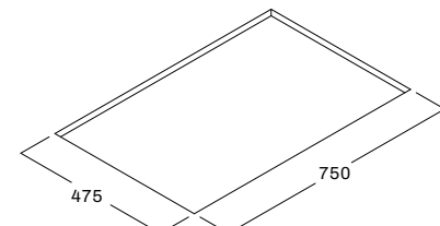
Montaje enrasado Flush mounting
