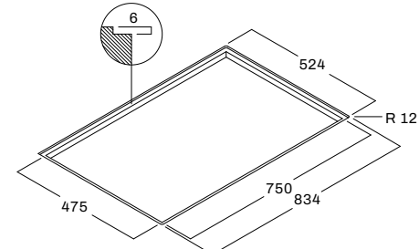
Montaje enrasado Flush mounting
