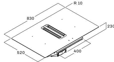
Montaje estándar Standard mounting
